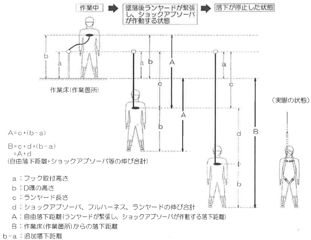
図1 フルハーネス型の落下距離等
